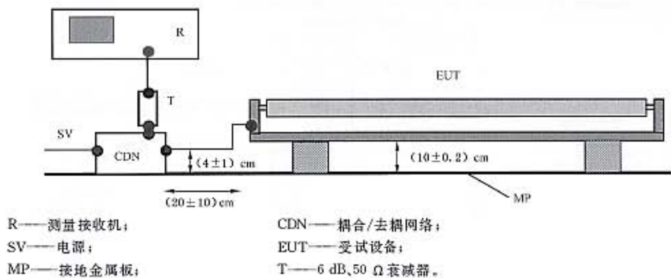
图 B.1 CDN 法的试验布置
